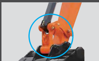
フック付き缶物先端プッシュ強化Aリンク
